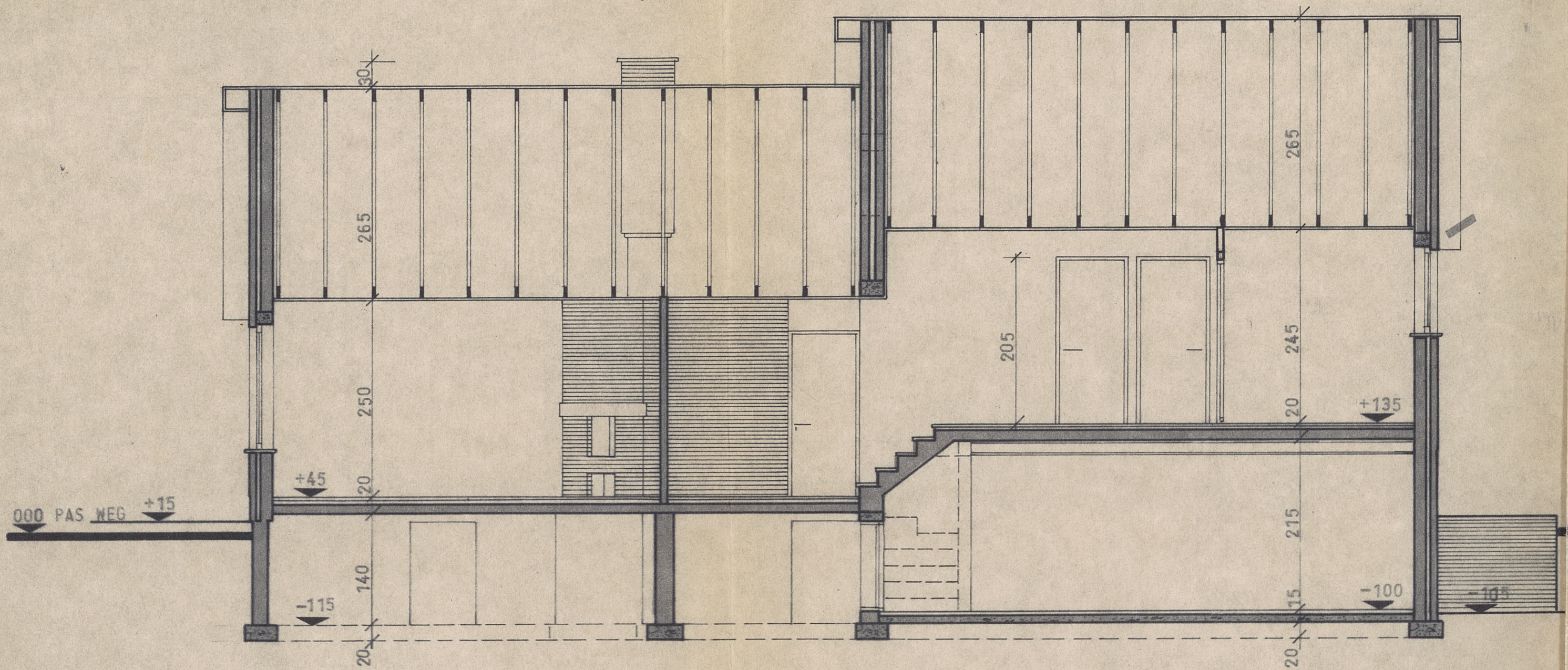
doorsnede a-b
